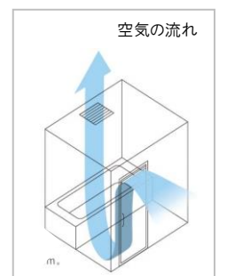
換気口をドアの上に。 お掃除性と換気性能を両立。
